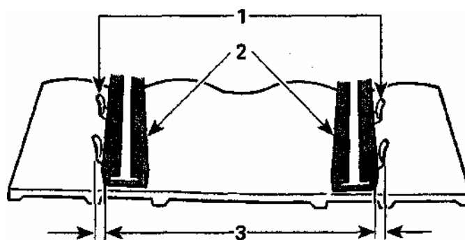
Рисунок 25 - Проверка симметричности положения гусеничной ленты
