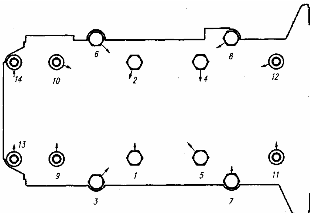
Рисунок 20 - Схема очередности затяжки болтов и винтов крепления
