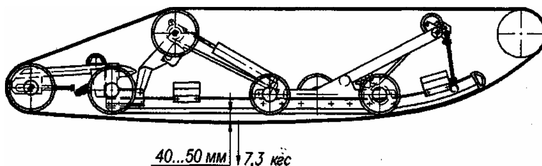
Рисунок 23 - Проверка натяжения гусеничной ленты
