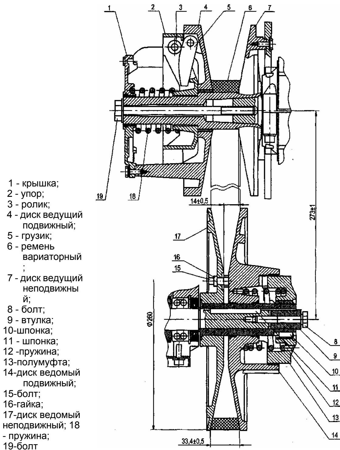
Рисунок 14 - Вариатор
