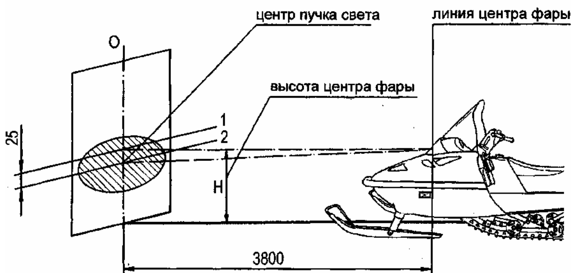
Рисунок 31 - Регулировка фары
