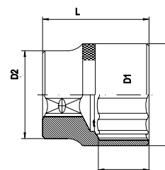
632 ГОЛОВКИ ДВЕНАДЦАТИГРАННЫЕ 3/4"
